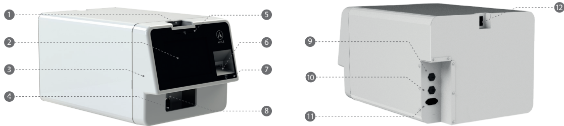
1. Entrée de pièces, 2. Écran tactile, 3. Porte de la machine, 4. Sortie de pièces, 5. Voyant indicateur pour le validateur de pièces actif, 6. Entrée et sortie de billets, 7. Voyant indicateur pour le validateur de billets actif, 8. Serrure cachée pour ouvrir la porte, 9. Bouton marche / arrêt de la machine (ON / OFF), 10. Port USB, 11. Connecteur câble réseau, 12. Connecteur câble d'alimentation
